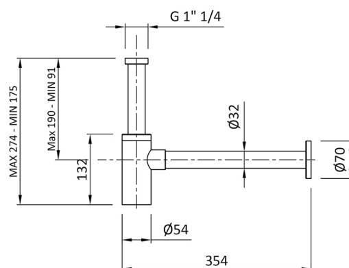
Dessin technique
